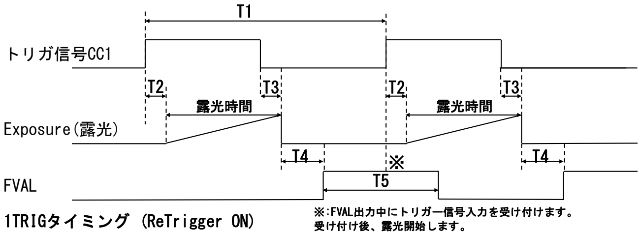
トリガーモード：1TRIG(トリガー幅シャッターモード) (PXC890B 高速版) ReTrigger ON 時
