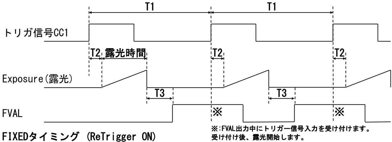
トリガモード : FIXED(固定シャッター) (PXC890B 高速版) ReTrigger ON 時
